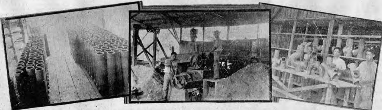
De izquierda a derecha: Alineados y simétricos, los tubos acaban de salir de la máquina. De allí se les traslada a las estanterías donde se "madurarán" para quemarse luego.—La máquina de amasar manejada por dos operarios.—Piezas vitrificadas en el momento en que las acomodan los empleados.
